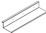
ELETTRIFICAZIONE ORIZZONTALE _HORIZONTAL CABLE MANAGEMENT
